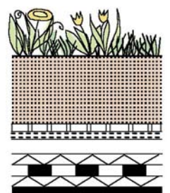
Intensive Dachbegrünung
